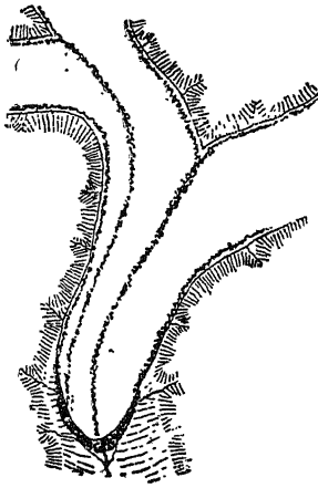
चित्र १८२—पार्श्व, मध्य और अन्तिम मोरेन्स
